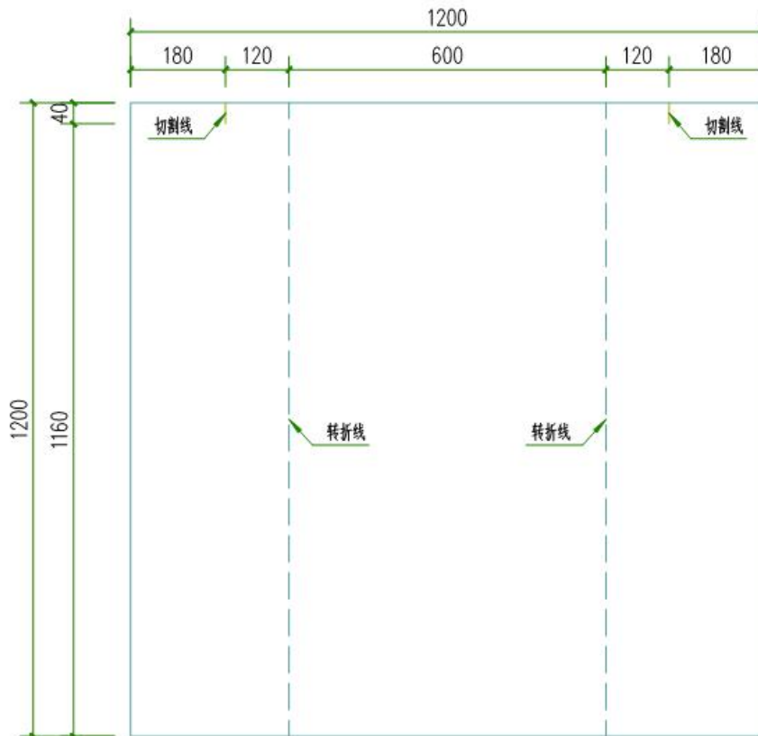
展示牌B件展开图
